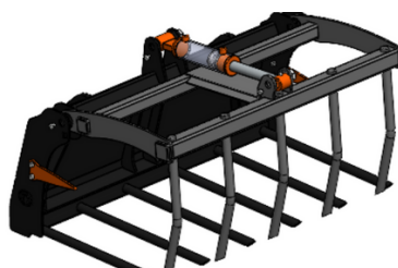
FORQUILHA PARA ESTRUME COM GRIFA
