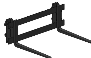
PORTA PALETES COM GARFOS AJUSTÁVEIS
