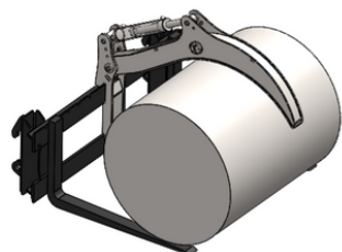
PORTA PALETES COM GRIFA PARA TOROS
